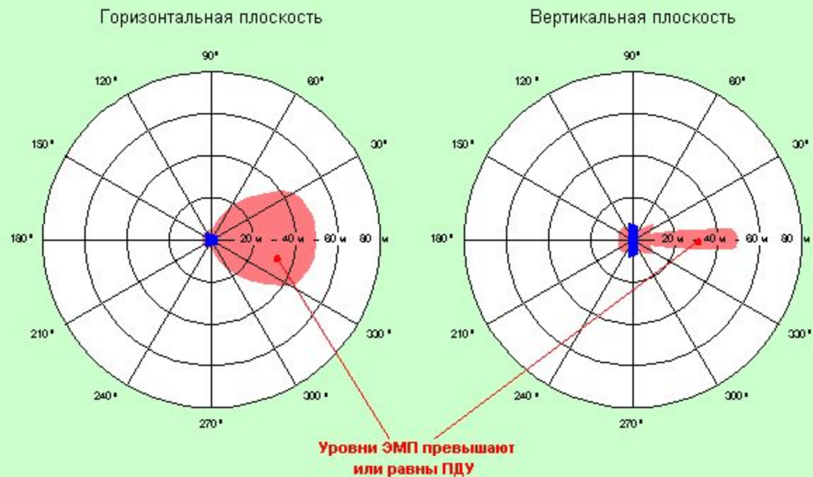
↑ Диаграмма направленности антенны типа "Оmnнi"
