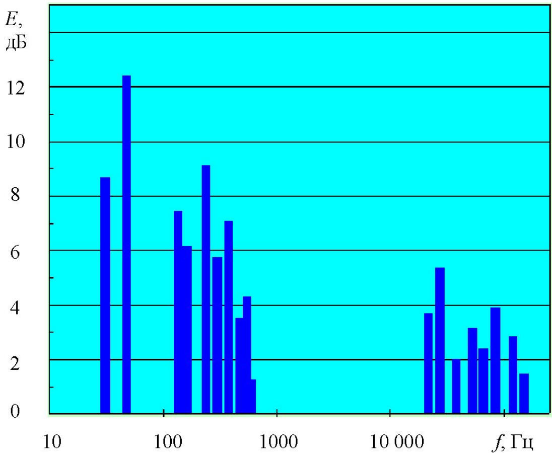
Спектральная характеристика излучения монитора в диапазоне 10 Гц...400 кГц
