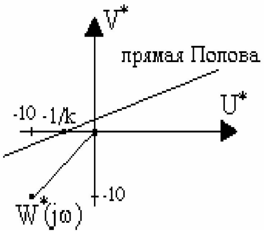
Видоизмененная частотная характеристика
