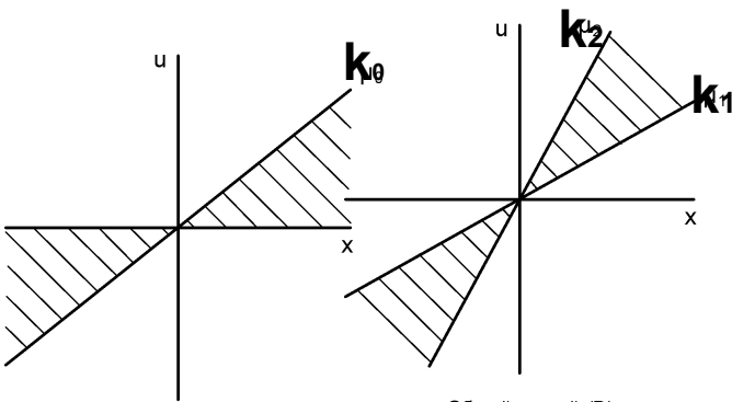
Общий случай (В) Сектор S[\mu_1, \mu_2]
