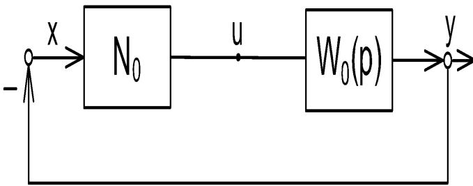
Базовый случай (А) Сектор S[\mu_0] \mu_1=0, \mu_2=\mu_0
