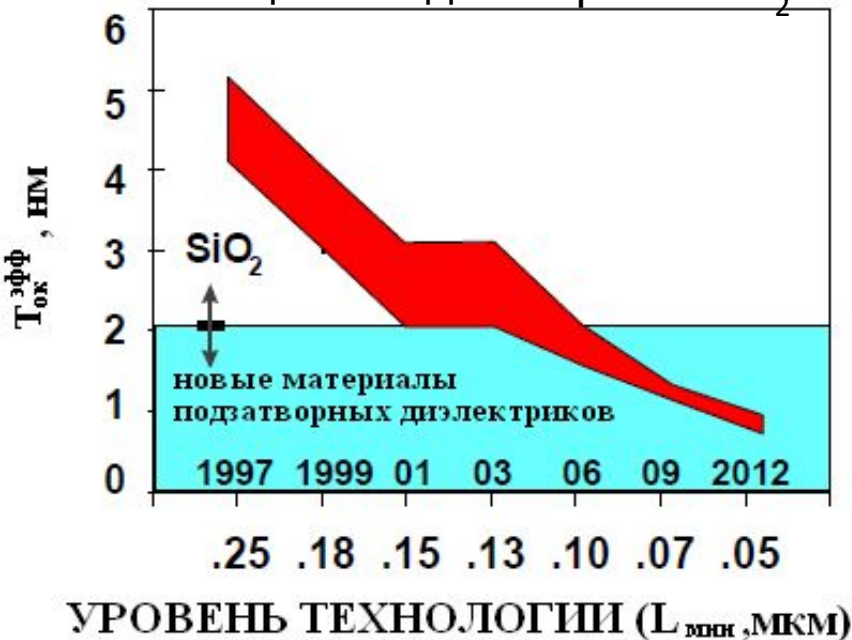
Прогноз масштабирования толщины подзатворного \text{SiO}_2
