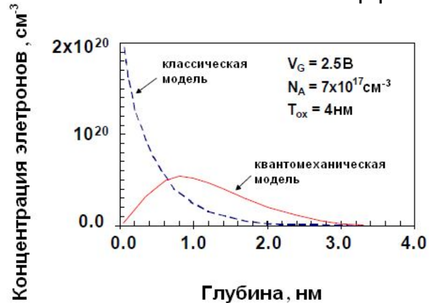
Кванто-механический эффект
