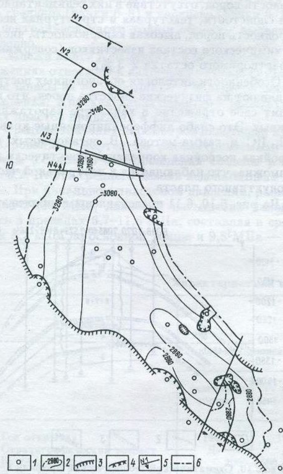
Рис. 6.8. Структурная карта по кровле пронизаемых песчаников основной толщи среднего девона: 1 — скважины; 2 — изогипсы; 3 — линия отсутствия песчаников I+II+III пачек основной толщи; 4 — линия замещения нефтенасыщенных песчаников I+II+III пачек основной толщи плотными породами; 5 — тектонические нарушения; 6 — внешний контур нефтеносности
