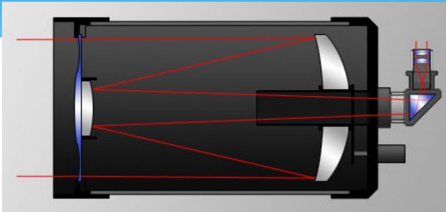
Телескоп Шмидта-Кассегрена
