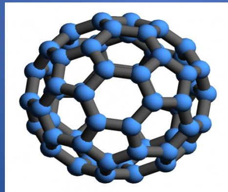
Атомы углерода
