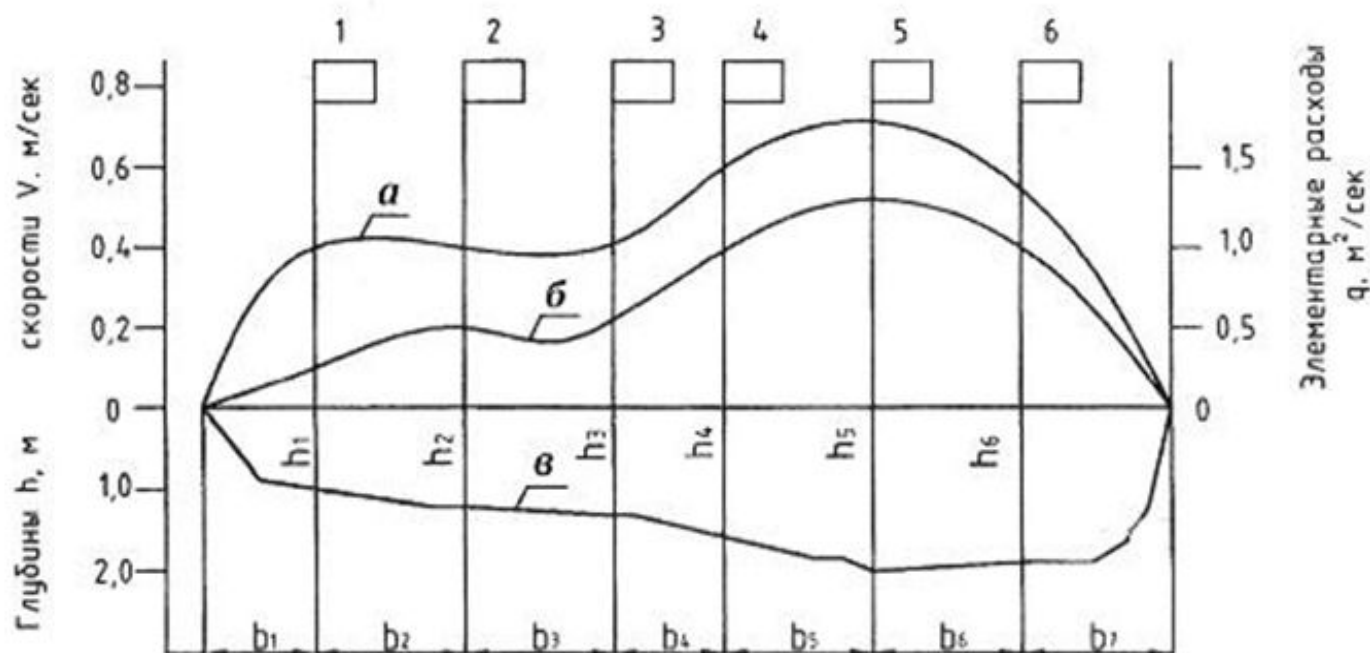
Рис. 9 . Вычисление расхода воды графическим способом:
