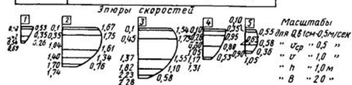
Рис. 79. Определение расхода воды графомеханическим способом
