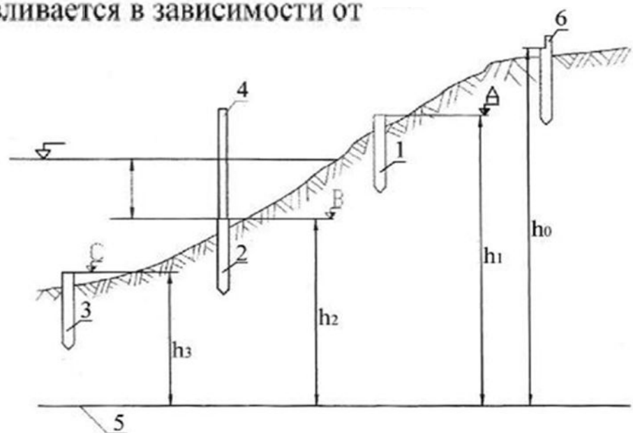
Рис. 2. Схема определения отметок уровня воды на свайном водомерном посту:
