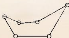
Конформация «ванны»
