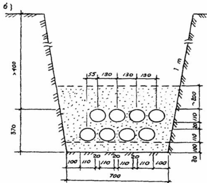
Рисунок 1 – Схемы расположения каналов связи из труб ТПЭ-КЭС в блоках
