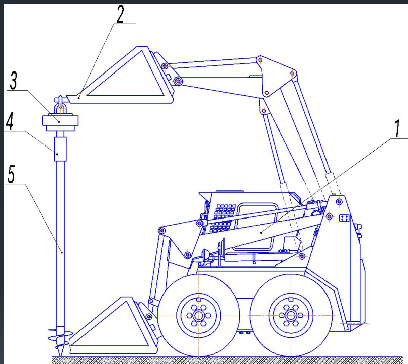
Рисунок 4 – Оборудование для погружения винтовых свай на погрузчике: 1 – погрузчик; 2 – подвеска оборудования; 3 – гидромотор; 4 – переходник; 5 – винтовая свая
