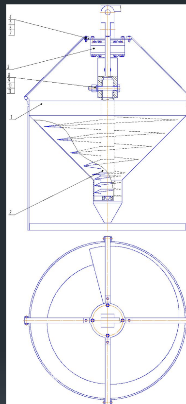
Рисунок 7 – Нагнетатель раствора в винтовые сваи: 1 – бак; 2 – шнек; 3 – вращатель; 4, 5, 6, 7 – крепёж бака к вращателю; 8, 9, 10, 11 – крепёж шнека к вращателю
