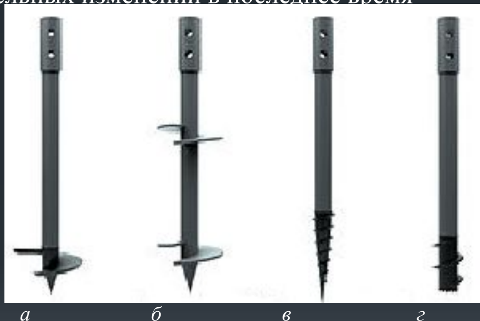
Рисунок 1 – Типы винтовых свай: а – широколопастная свая с одной лопастью; б – широколопастная свая с двумя и более лопастями; в – узколопастная многовитковая свая; г – свая для вечномёрзлых грунтов
