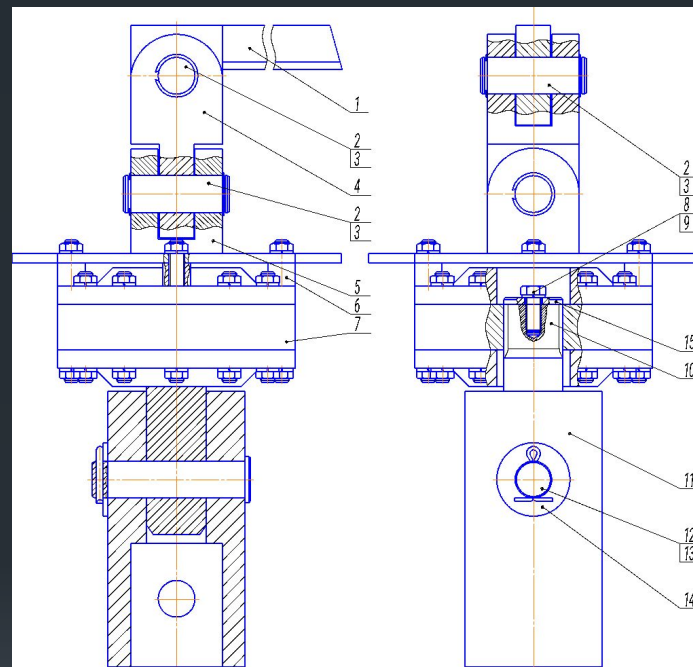
Рисунок 5 – Вращатель: 1 – верхний крепеж; 2 – ось; 3 – стопорное кольцо; 4 – ось; 5 – нижний крепеж; 6 – втулка; 7 – гидромотор; 8,9 – болтовой крепеж; 10 – вал; 11 – переходник; 12 – палец; 13 – шплинт; 14 – шайба
