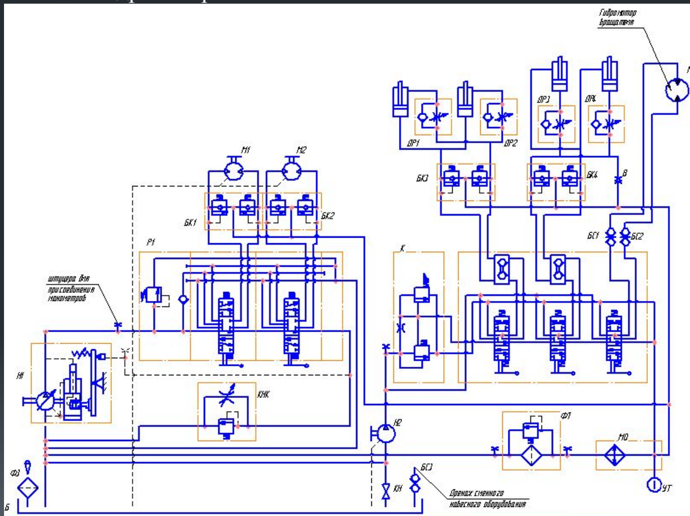
Рисунок 8 – Гидравлическая схема погрузчика с изменениями для привода вращателя
