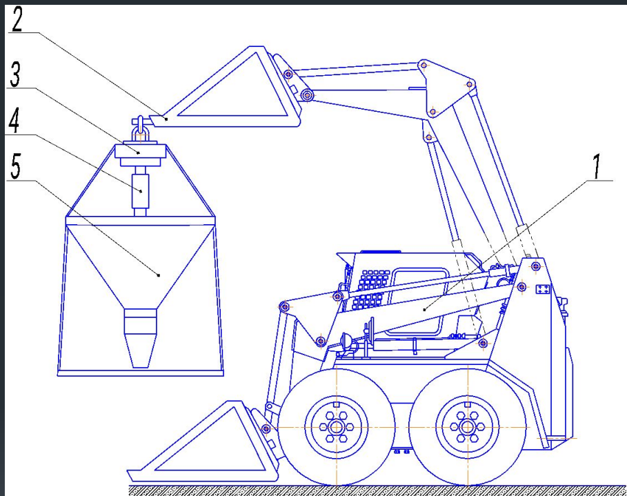
Рисунок 6 – Оборудование для заполнения раствором винтовых свай на погрузчике: 1 – погрузчик; 2 – подвеска оборудования; 3 – гидромотор; 4 – переходник; 5 – нагнетатель раствора
