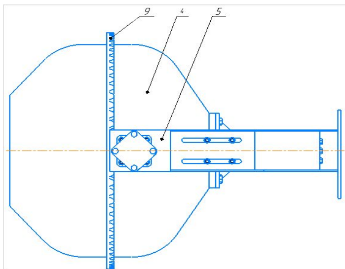
Рисунок 2 – Бетоносмеситель: 1-рама, 2-опорный узел, 3-косынка фланца, 4-бочка, 5-крепление гидромотора, 6-площадка, 7-шестерня гидромотора, 8-гидромотор, 9-венец
