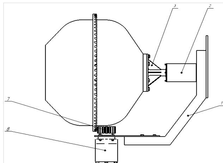
Рисунок 2 – Бетоносмеситель: 1-рама, 2-опорный узел, 3-косынка фланца, 4-бочка, 5-крепление гидромотора, 6-площадка, 7-шестерня гидромотора, 8-гидромотор, 9-венец
