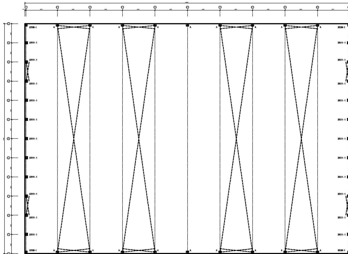
План здания
