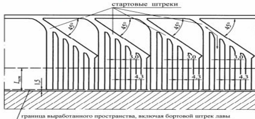
б) с расположением стартовых штреков под углом 45^\circ , а очистных ходов под углом 90^\circ к границе отработки.
