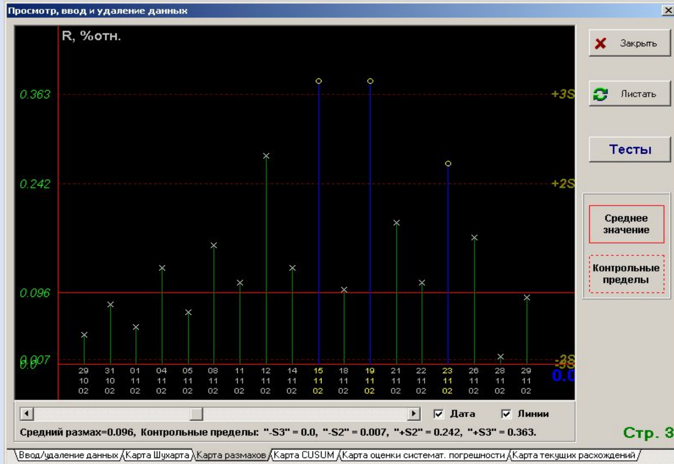
Контрольная карта Шухарта (размахов)
