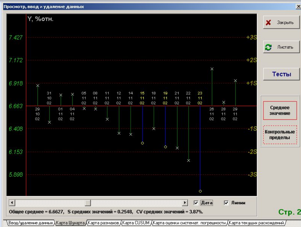
Контрольная карта Шухарта (средних значений)
