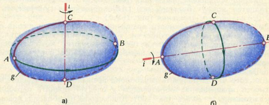
Рис. 159 Эллипсоид: а — сжатый, б — вытянутый
