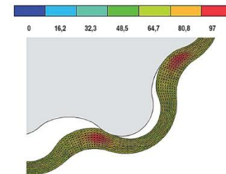
Разогрев обкладки статора R-Wall RS172N645W, max t = 96°C
