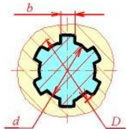
Сечение прямобочного шлицевого соединения
