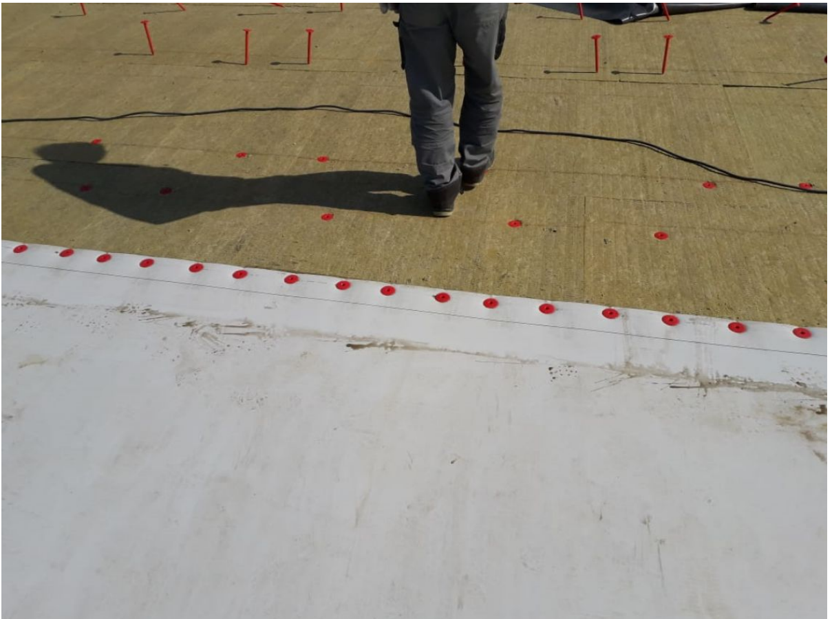
Монтаж пирога кровли / Installation of roof pie
