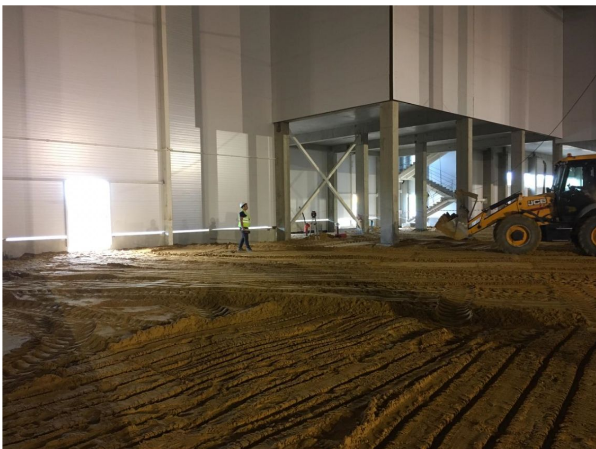
Разработка грунта под плиту пола / Excavation of soil under the floor slab
