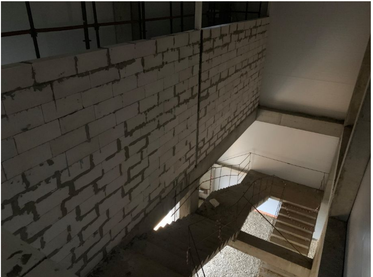
Монтаж стен из бетонных блоков / Installation of concrete block walls
