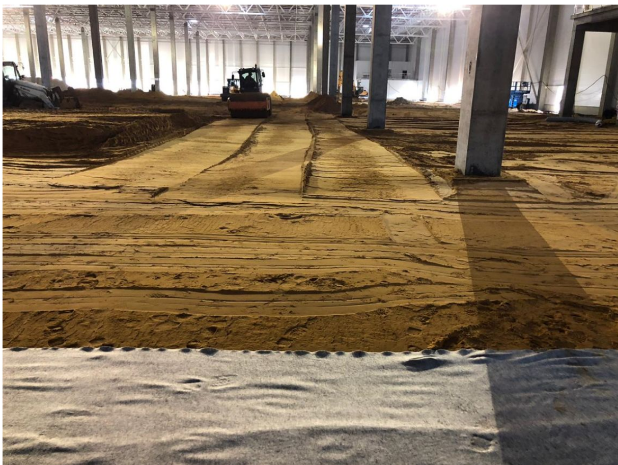
Устройство песчаного основания под плиту пола/ Making sand foundations for the floor slab
