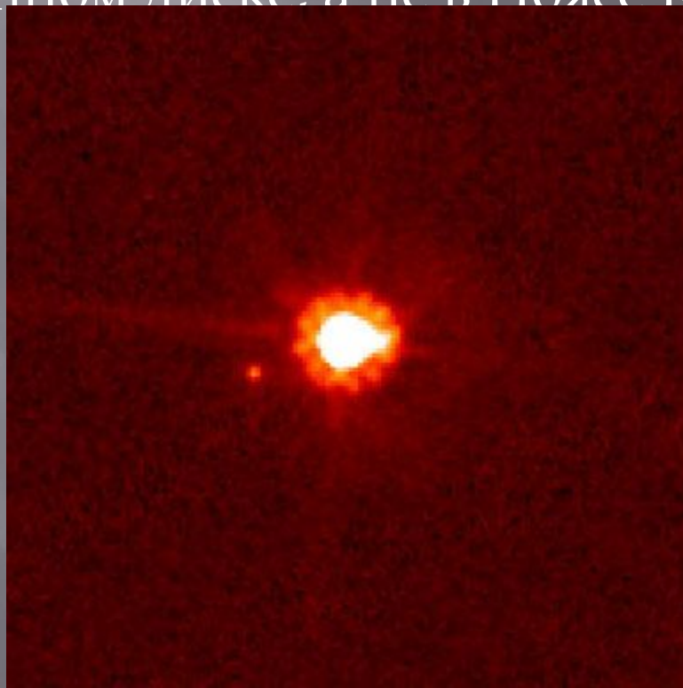
Самое качественное настоящее изображение Эриды
