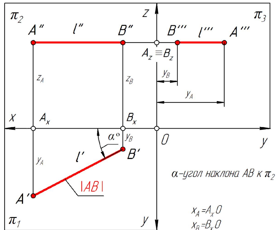
Горизонтальная прямая
