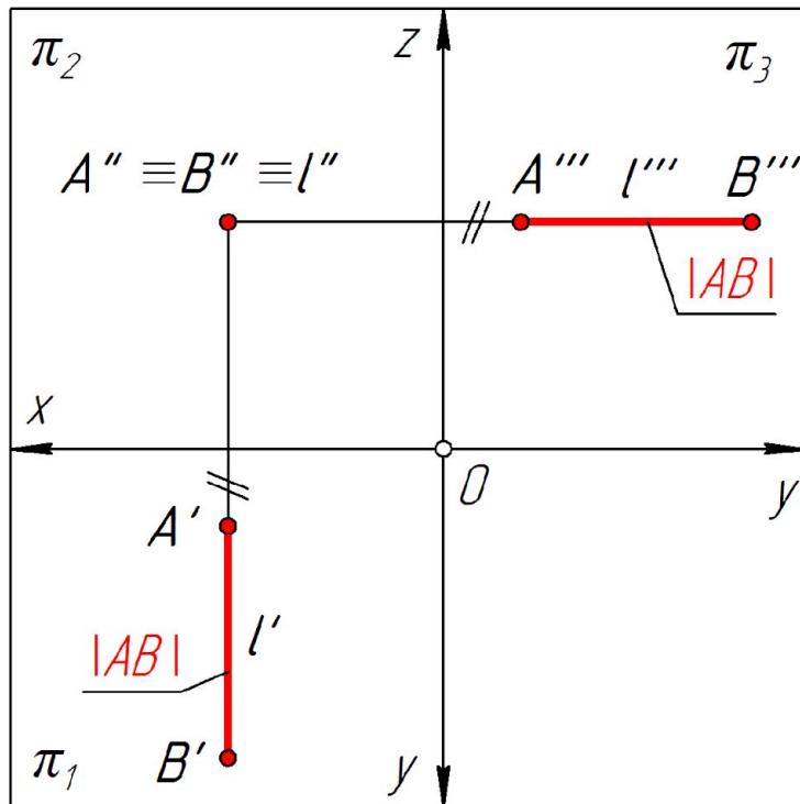
Фронтально-проецирующая прямая
