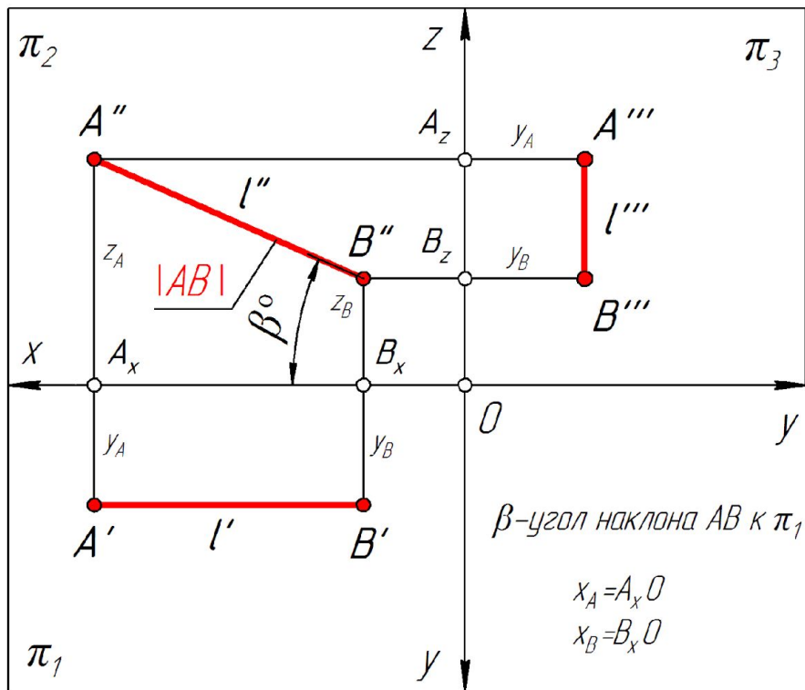
Фронтальная прямая
