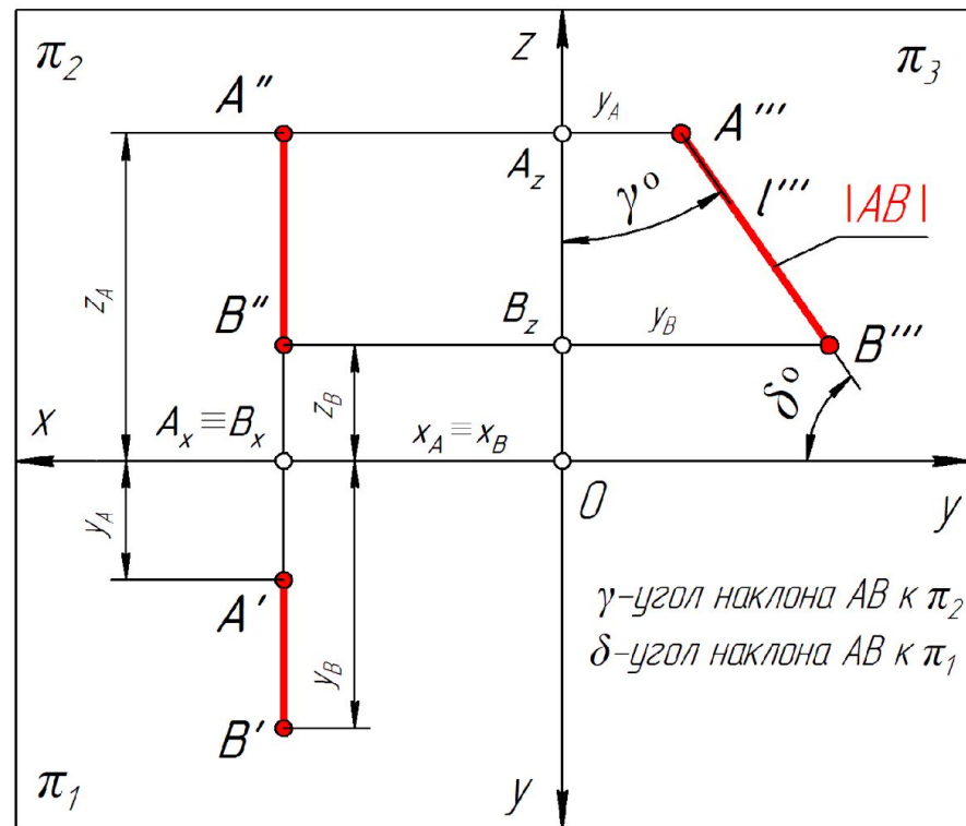
Профильная прямая
