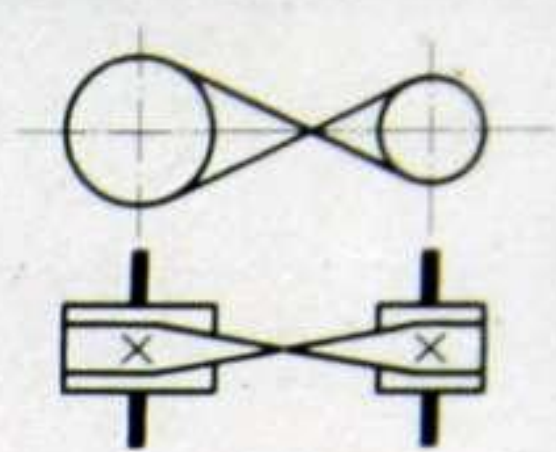
Перекрестная
