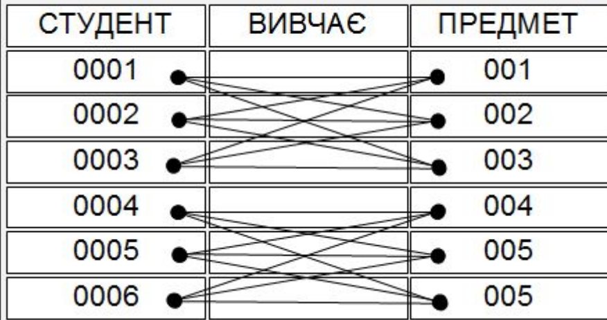
Діаграма ER-екземплярів
