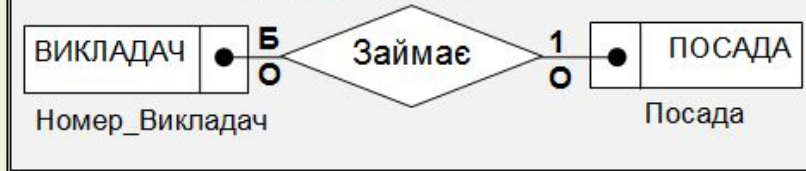
Діаграма ER-типів
