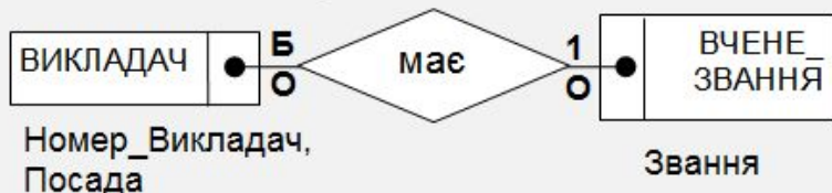
Діаграма ER-типів
