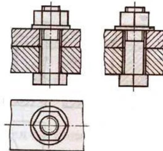
Болтовое соединение
