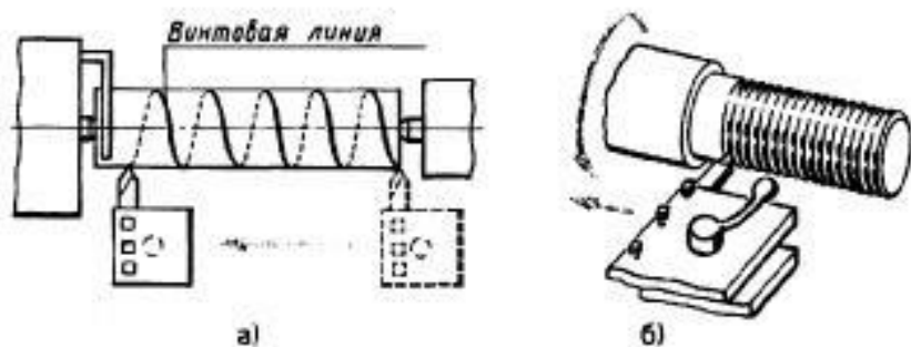
Рис. 205. Нарезание резьбы
