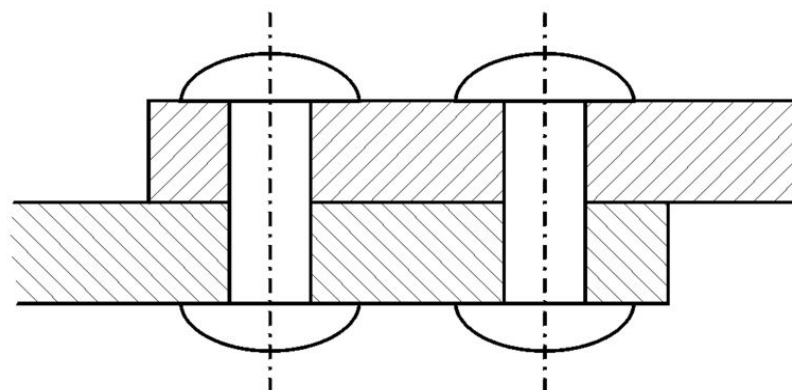
Соединение заклепками
