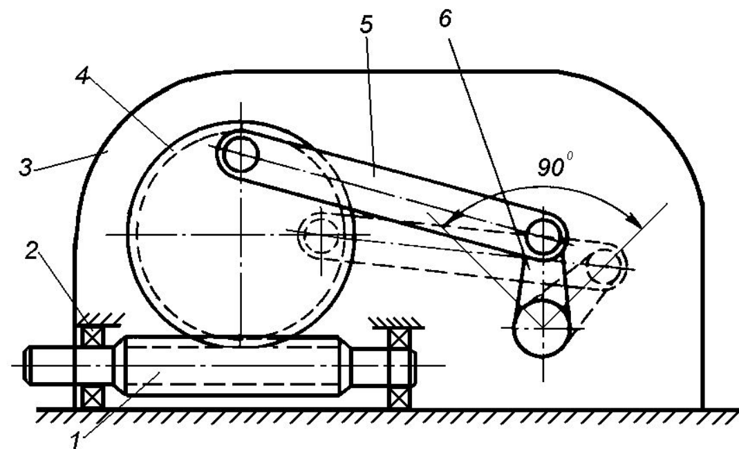
Редуктор привода
