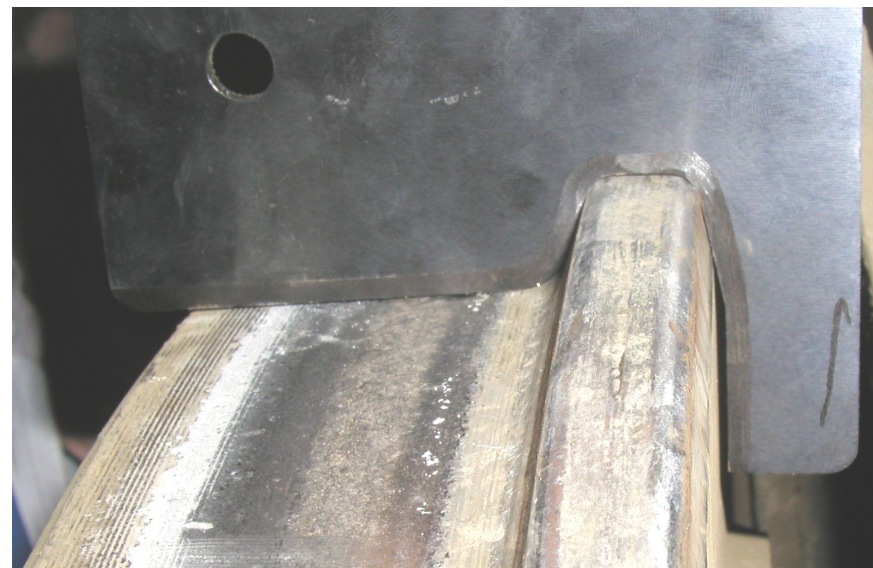
Проверка профиля колеса с помощью шаблона
