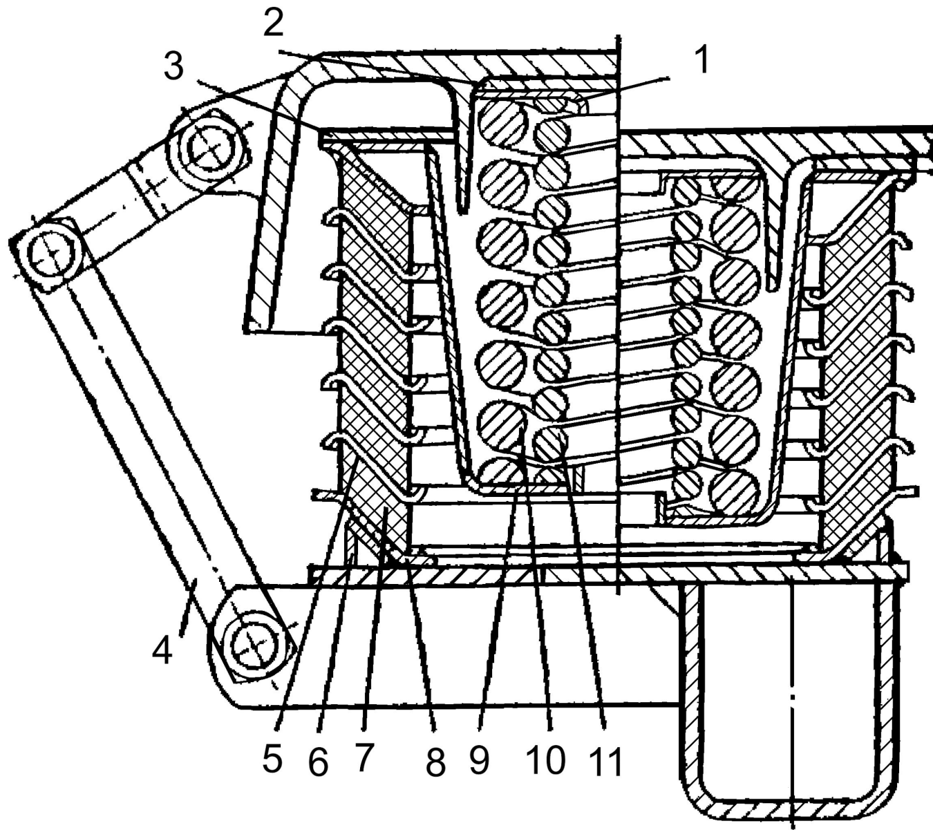
Рессорное подвешивание
