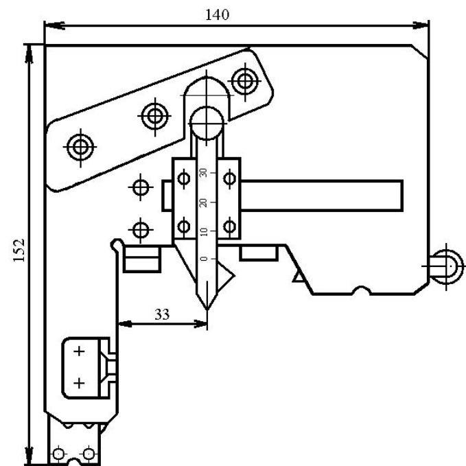
Ребордомер
