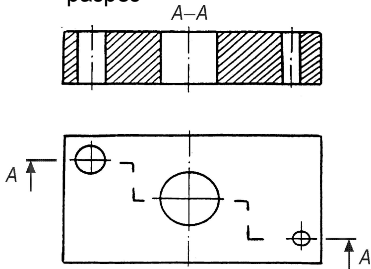
Ступенчатый разрез
