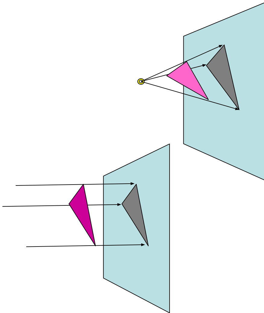
Метод прямоугольного параллельного проецирования
