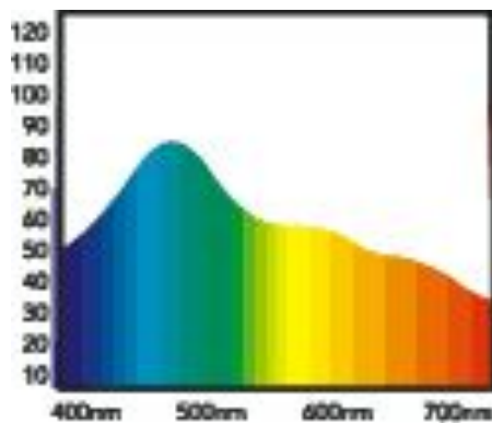
Спектр дневного света
