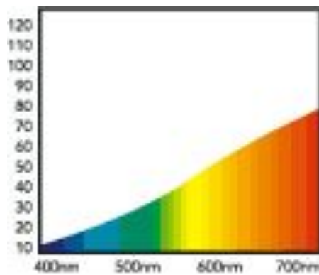
Спектр света лампы накаливания
