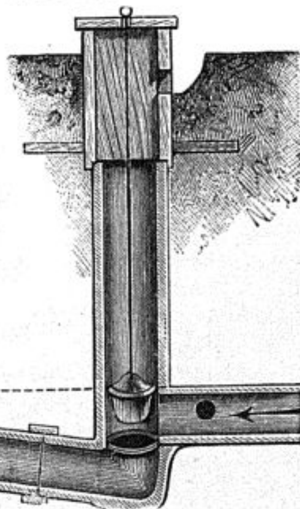
11. Клапанъ Петерсена въ вертикальномъ затворомъ.
