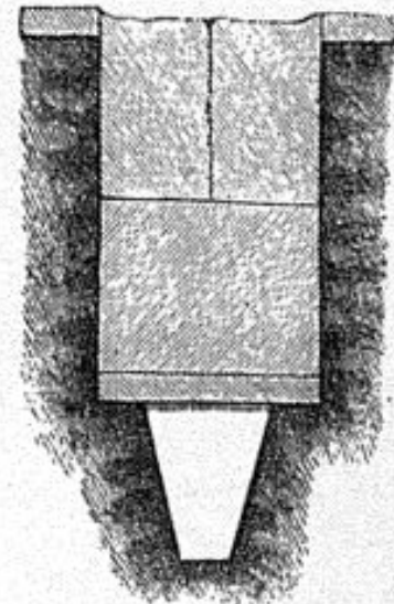
6. Дренажъ въ торфянистомъ грунтѣ.
