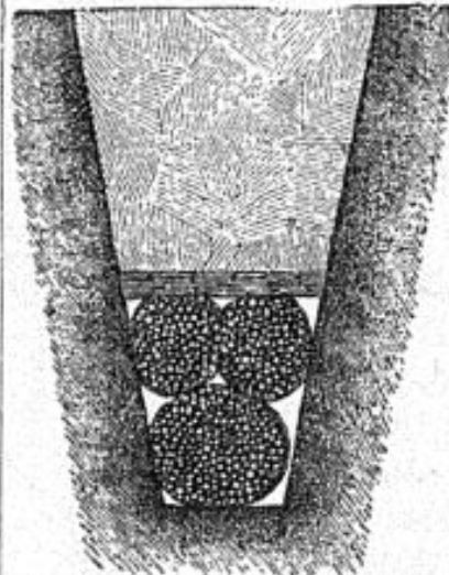
4. Фашинный дренажъ.
