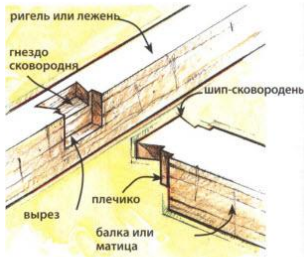
Рис. 32. Соединения деталей: 1 — сквороднем (а — брус, б — бревно); 2 — полусквороднем
