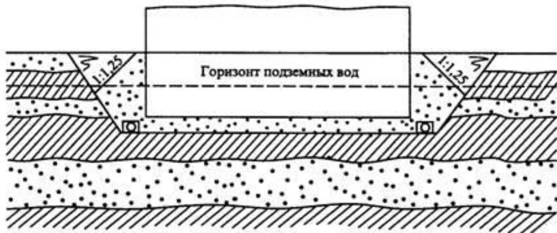
Разрез А-А
