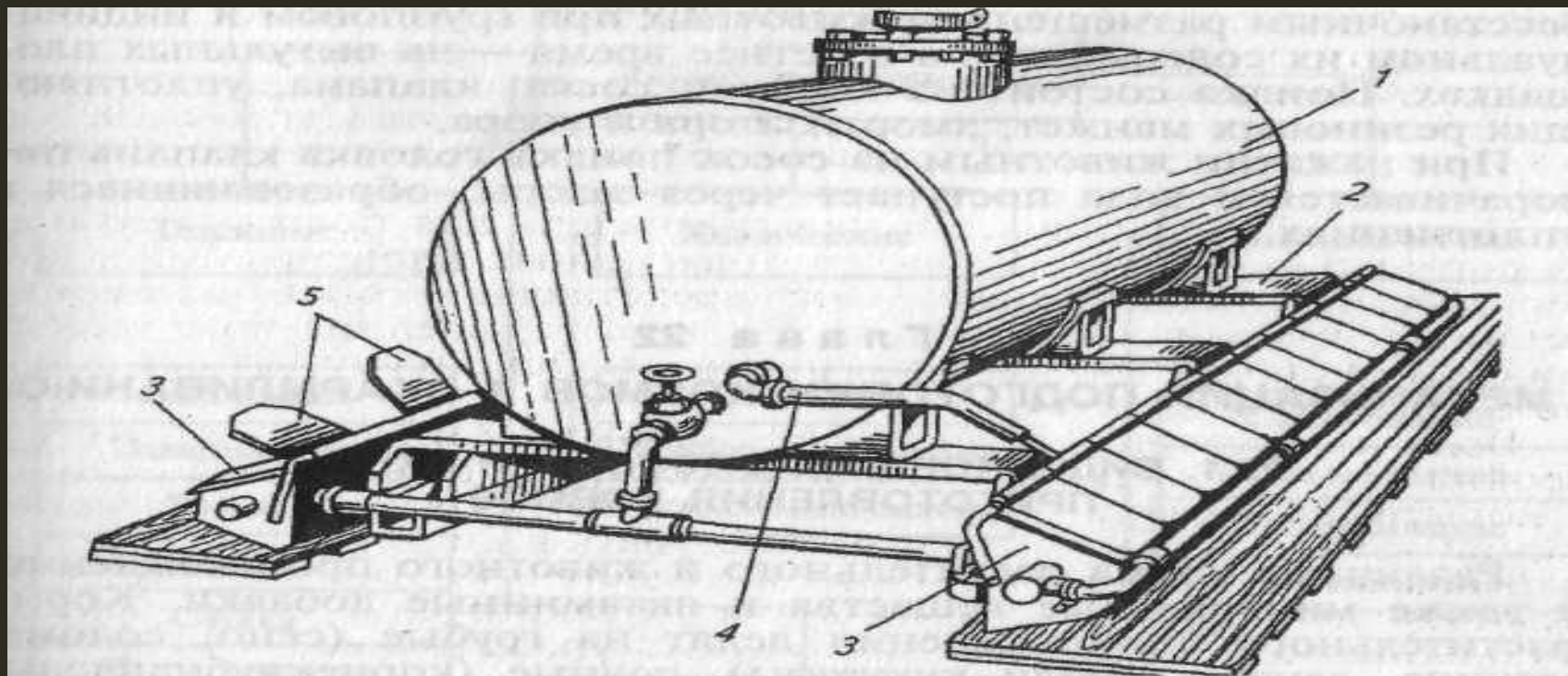
Рис. 21.7. Групповая автопоилка АГС-24:
