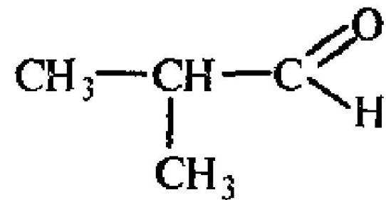
2-метилпропаналь
