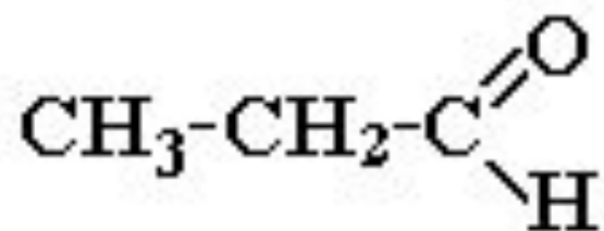
пропаналь
