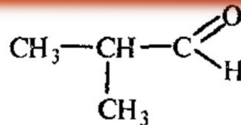
2-метилпропаналь
