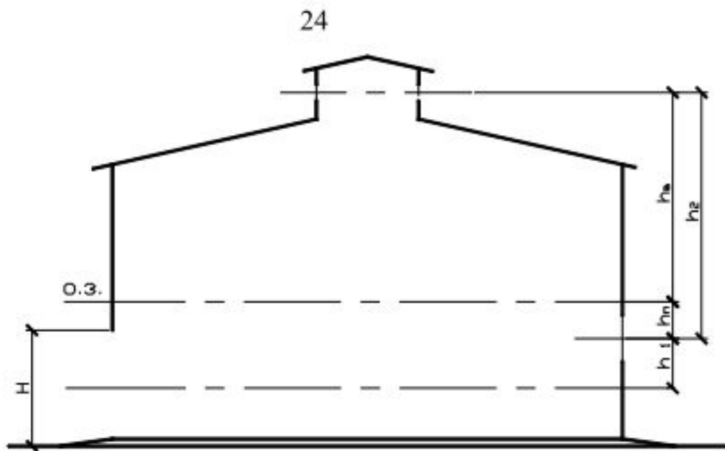
Здание с фонарями и закрытыми аэрационными фрамугами
