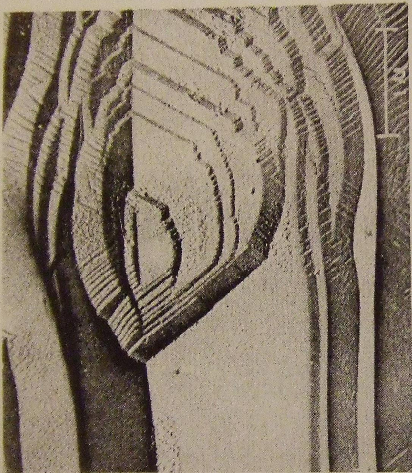
Struktura krystalu bariem titanátu v elektrovém mikroskopu
