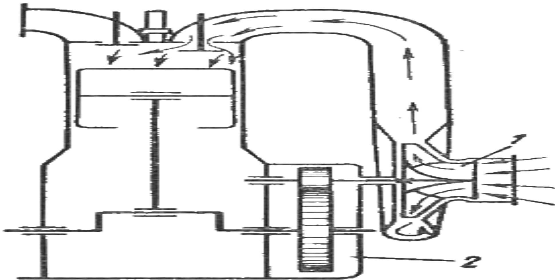
Фиг. 76. Схема наддува с механическим приводом: 1 — центробежный нагнетатель; 2 — зубчатая передача.
