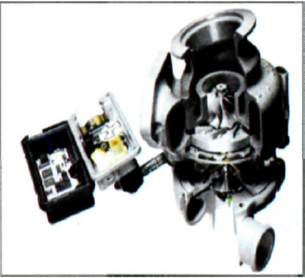
Рис. 2.108. Внешний вид турбокомпрессора с изменяемой геометрией
