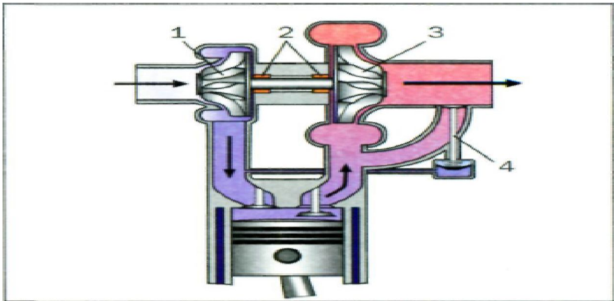
Рис. 2.105. Регулирование наддува: 1 — колесо компрессора; 2 — подшипники ротора; 3 — колесо турбины; 4 — перепускной клапан
