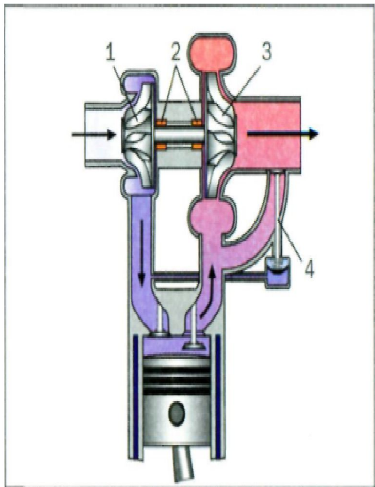
Рис. 2.105. Регулирование наддува: 1 — колесо компрессора; 2 — подшипники ротора; 3 — колесо турбины; 4 — перепускной клапан
