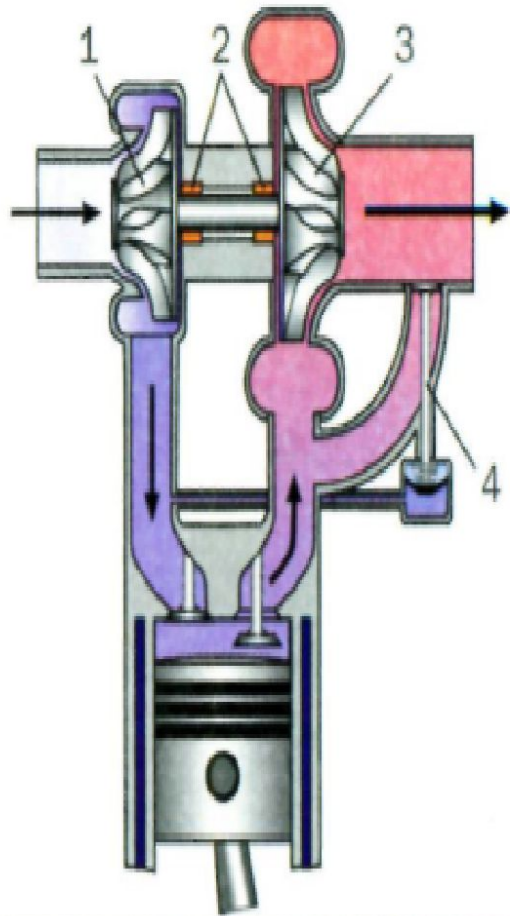
Рис. 2.105. Регулирование наддува: 1 — колесо компрессора; 2 — подшипники ротора; 3 — колесо турбины; 4 — перепускной клапан
