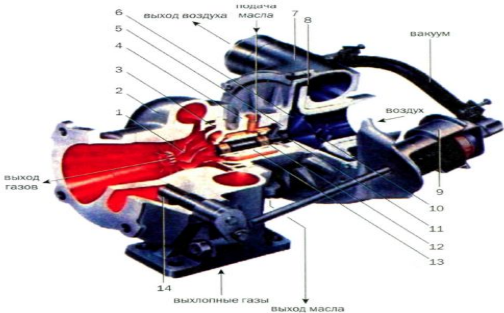
Рис. 2.106. Турбокомпрессор Garrett: 1 — лопатки турбины; 2 — корпус турбины; 3 — тепловая защита; 4 — корпус подшипников; 5 — упор; 6 — защитная пластина; 7 — корпус компрессора; 8 — диффузор; 9 — клапан; 10 — насос компрессора; 11 — уплотнение; 12 — подшипник; 13 — втулка подшипника; 14 — заслонка
