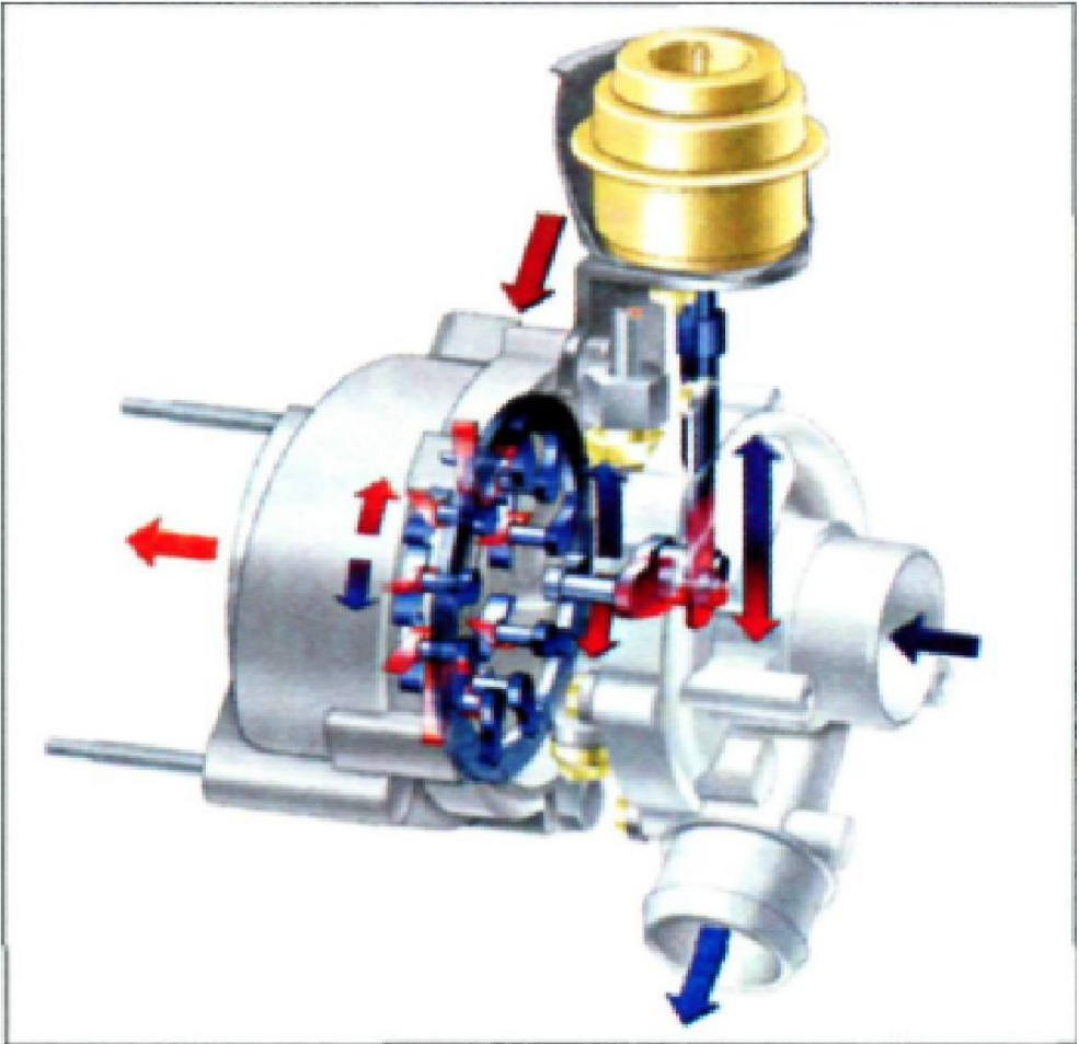
Рис. 2.107. Схема работы турбокомпрессора с изменяемой геометрией
