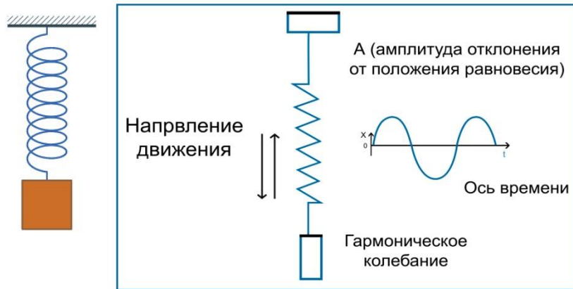
Простейшее гармоническое колебание
