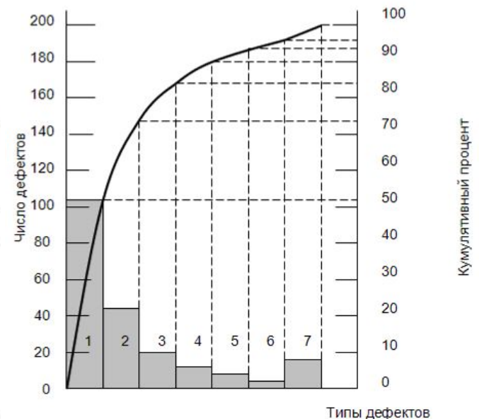
Рисунок 6.1 - Диаграмма Парето по типам дефектов деталей 1 – деформация; 2 - царапины; 3 – раковины; 4 – трещины; 5 – пятна; 6 – разрыв; 7 – прочие.
