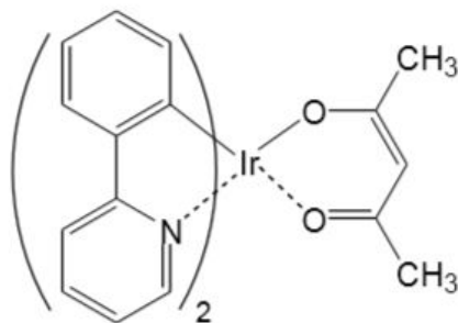
ppy 2 Ir(acac)
