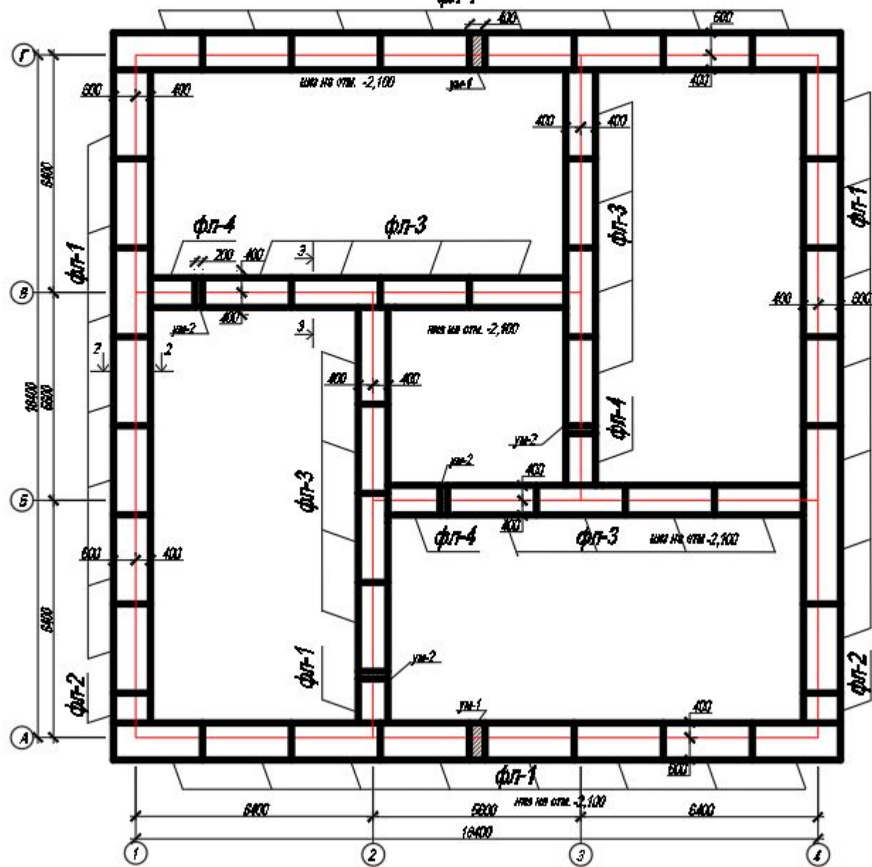
схема расположения подушек фундамента ФЛ-1
