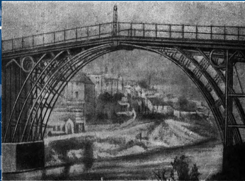
112. Чугунный арочный мост на р. Северн у Брозлея. Арх. Рейнольдс и Дерби, 1776—1779 гг. Пролет 30,6 м, стрелка 12,8 м
