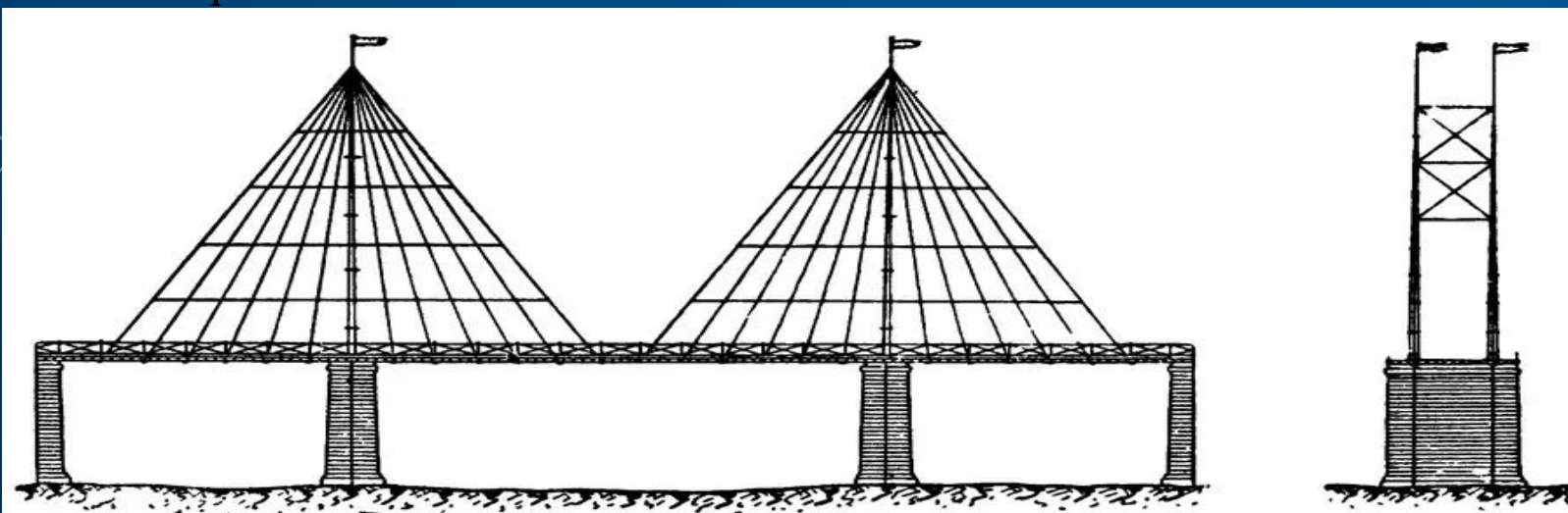
113. Проект вантового моста. Инж. Пойе, 1790 г.
