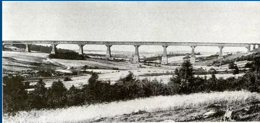
Веребьинский мост на линии Петербург—Москва. Автор проекта Д. И. Журавский. 1851
