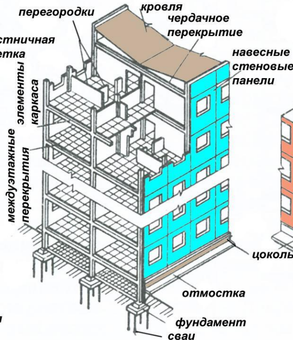
каркасно-панельное здание
