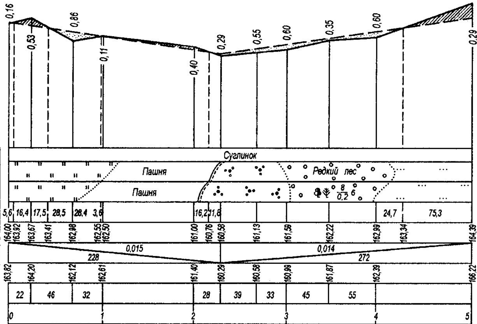
Продольный профиль
