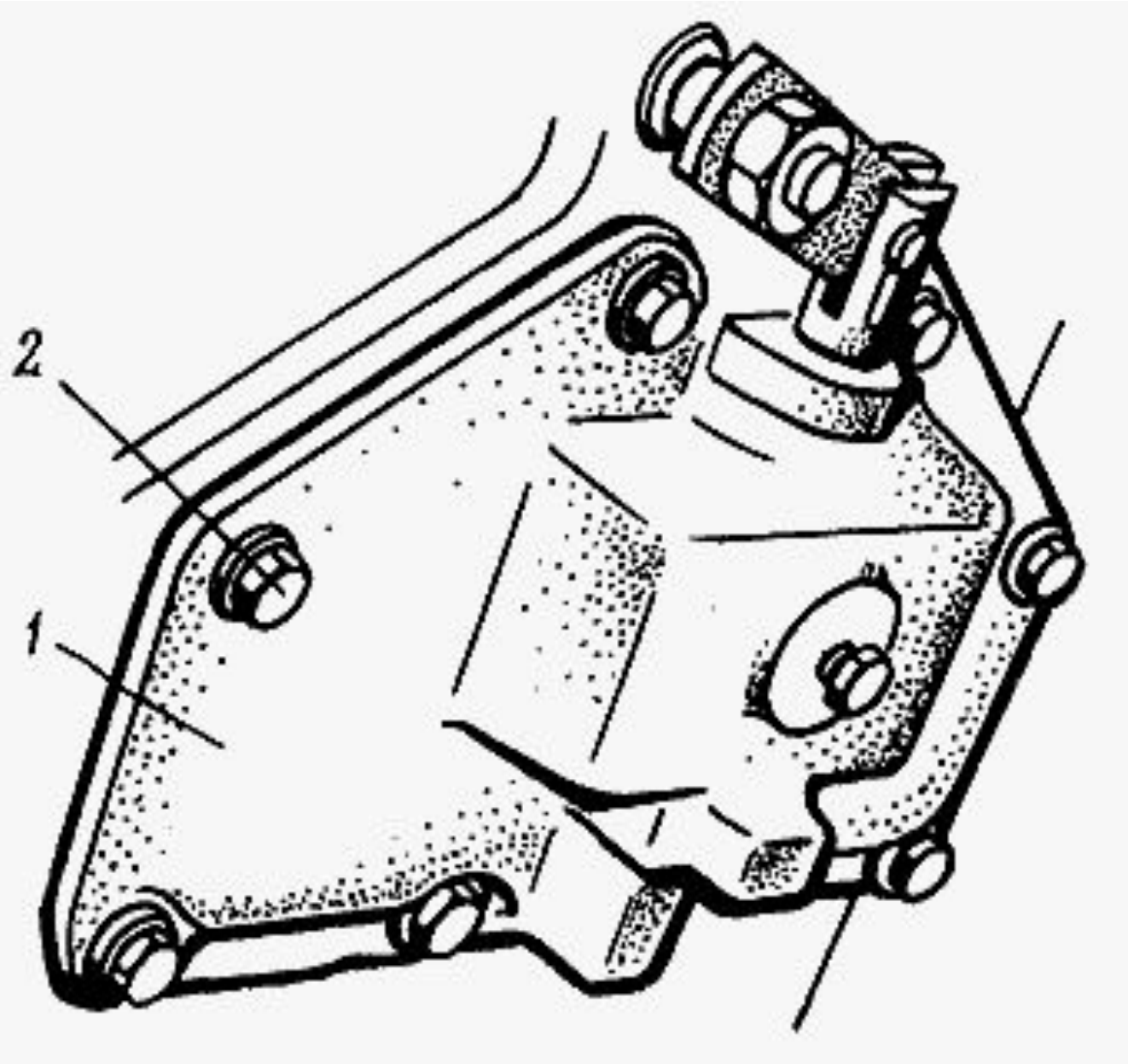
Рис.6. Снятие нижней крышки в сборе с вилкой переключения ступеней привода ВОМ МТЗ-80, МТЗ-82
