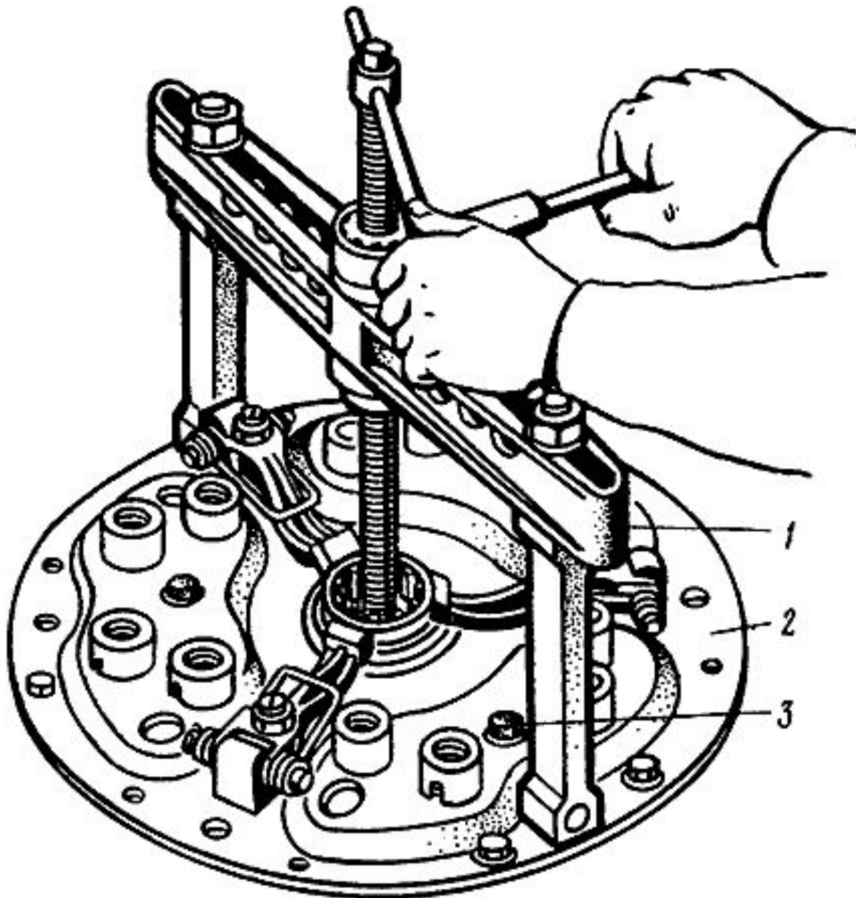
Рис. 2.5.2. Разборка опорного и нажимного дисков
