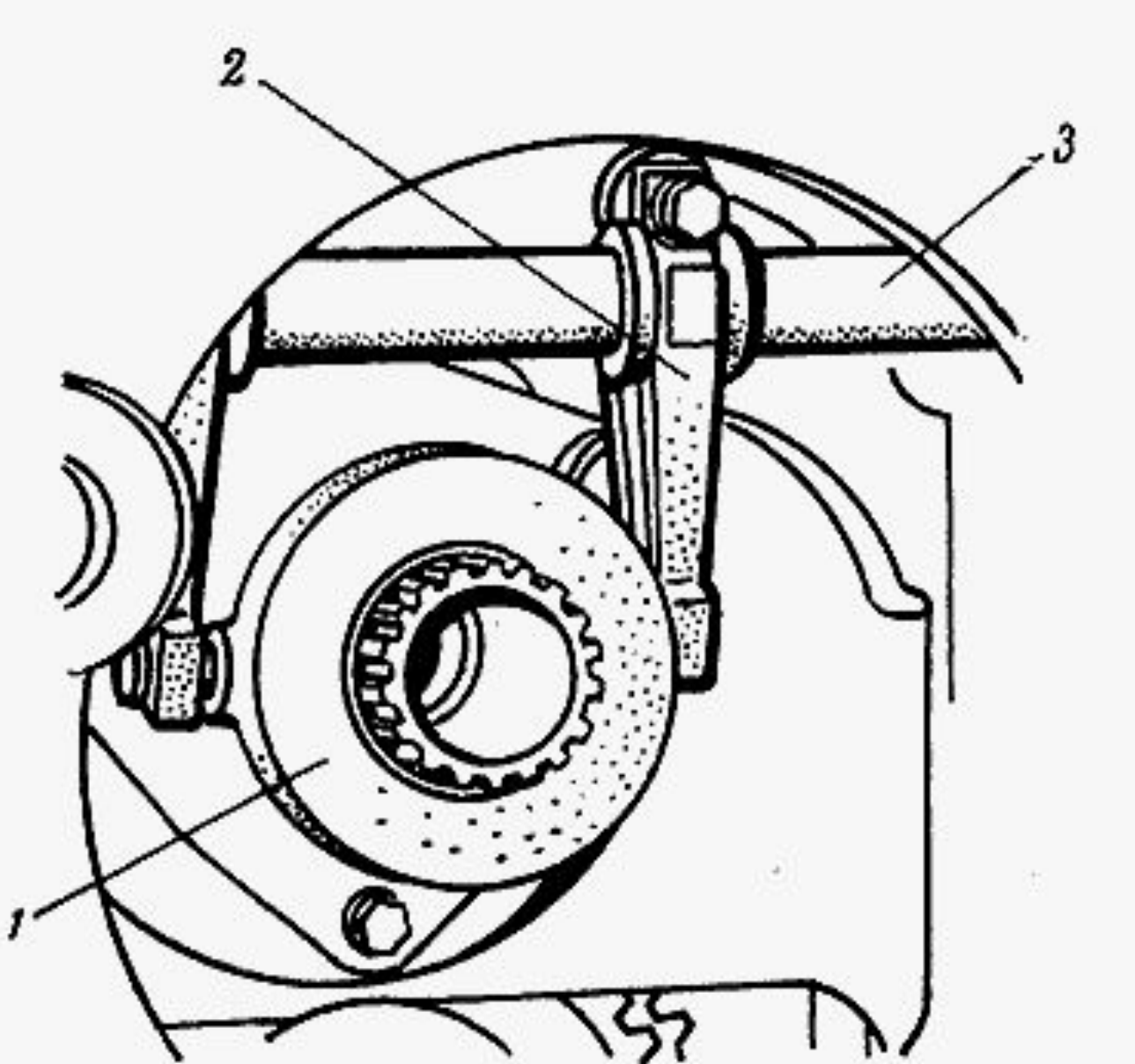
Рис. 5. Снятие упорного подшипника, отводки, вилок включения и вала вилок сцепления МТЗ-80, МТЗ-82
