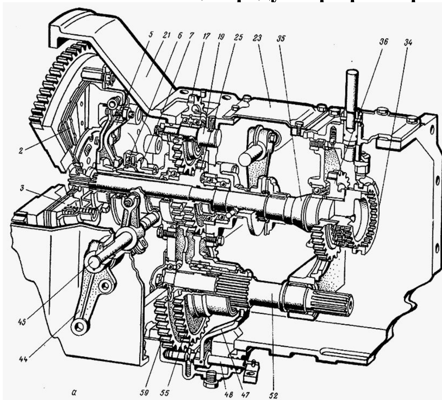
Рис.3. Сцепление и понижающий редуктор трактора МТЗ-80, МТЗ-82
