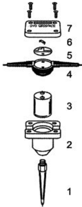
Схема комплектации электродинамического сейсмоприемника
