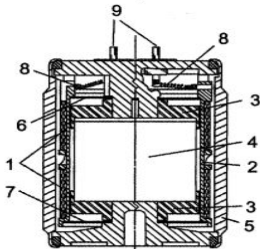
Разрез чувствительного элемента
