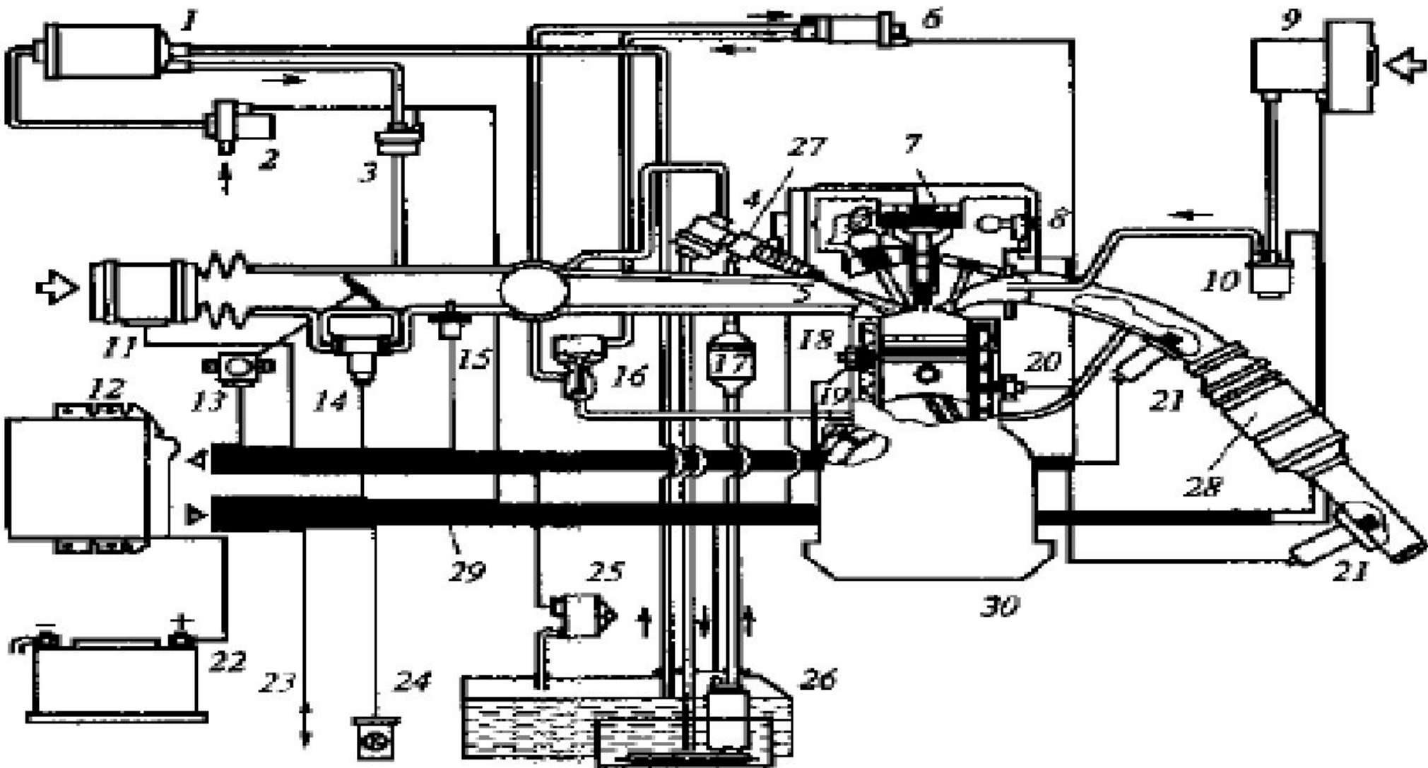
Рис. 23.2. Компьютерная система управления работой бензинового двигателя:
