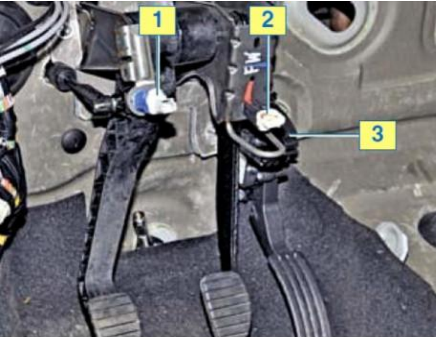
1 – датчик положения педали сцепления; 2 – выключатель сигнала торможения; 3 – модуль педали газа
