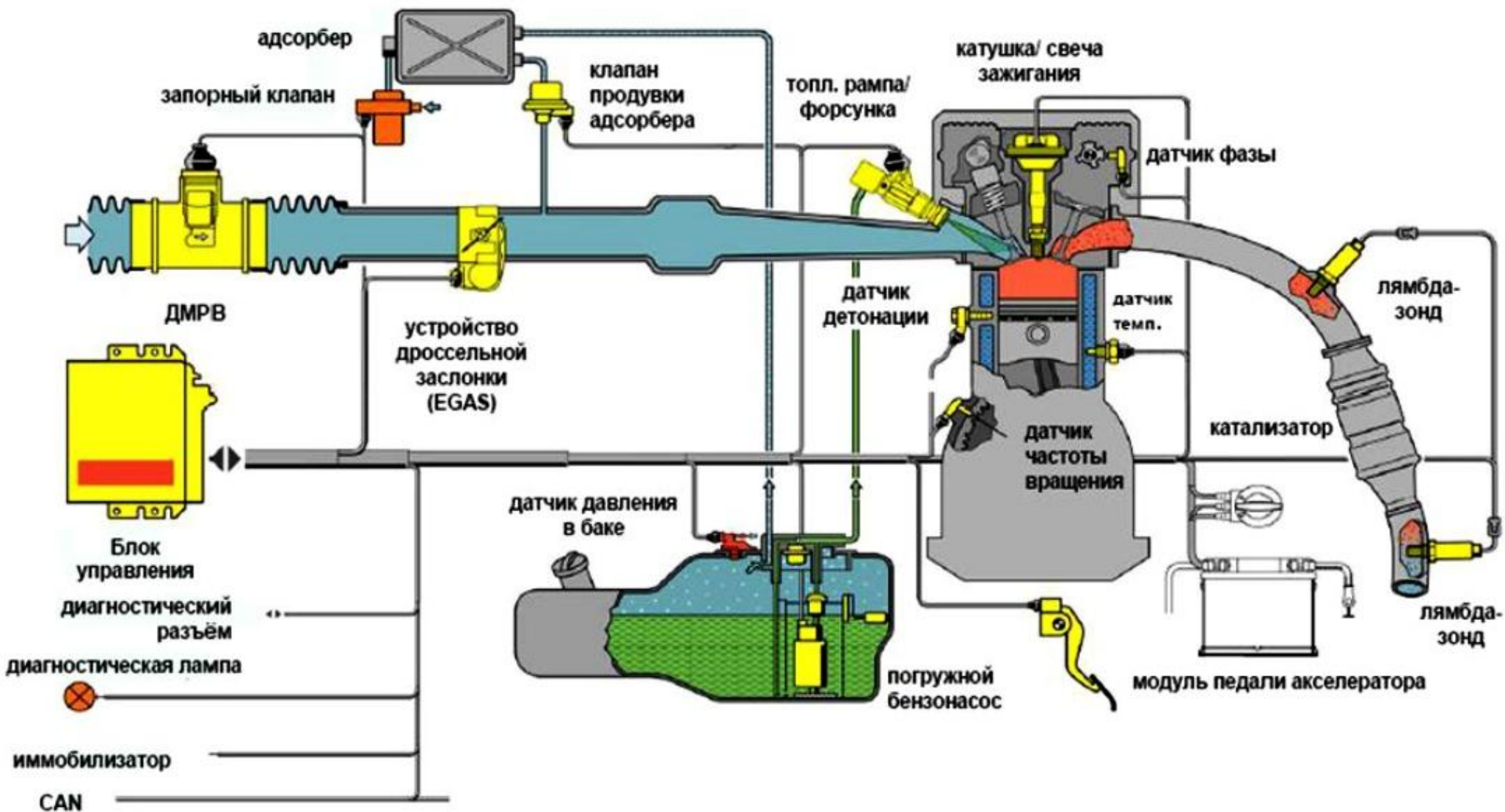
Принципиальная схема системы питания и управления
