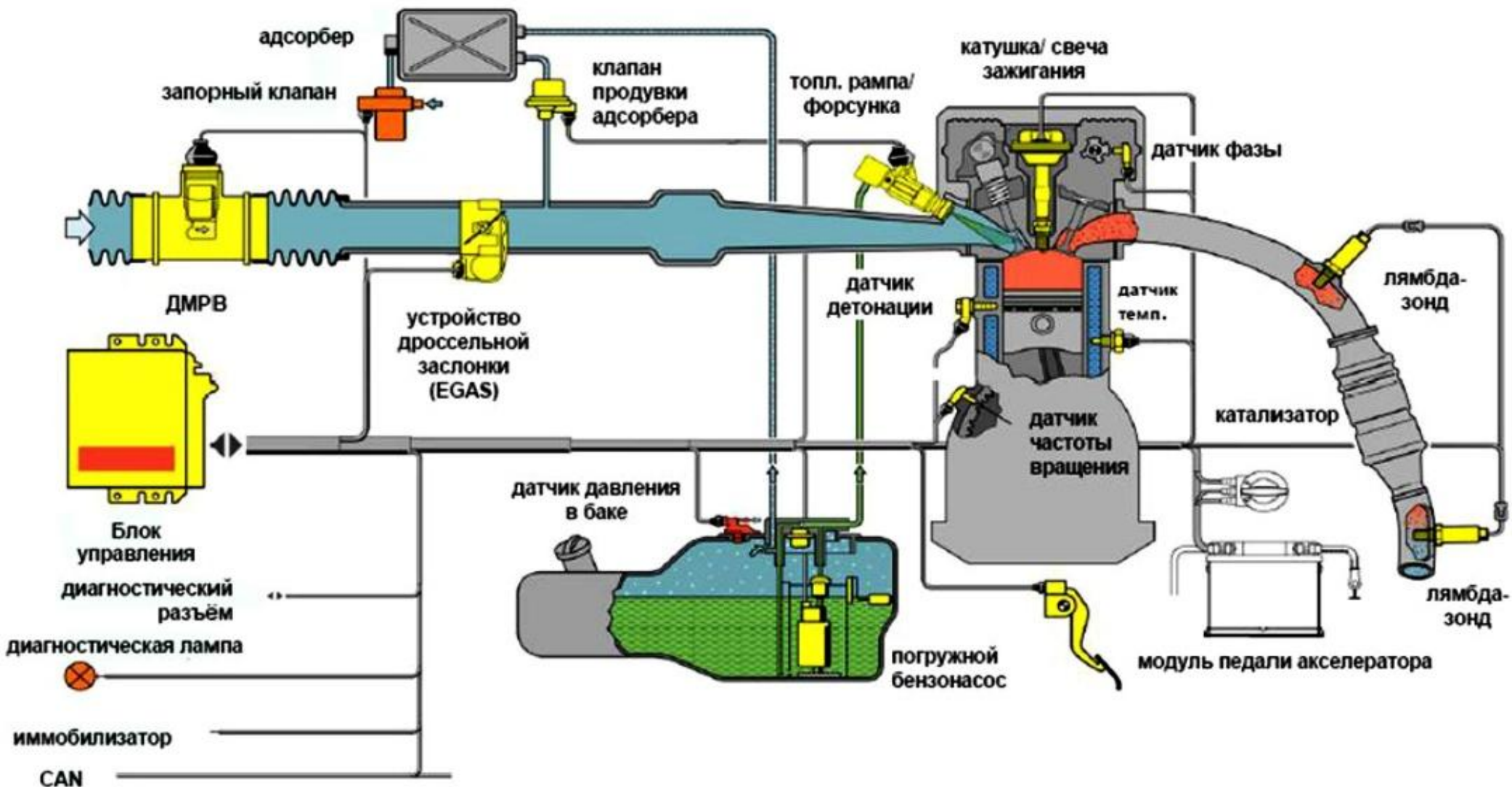
Принципиальная схема системы питания и управления
