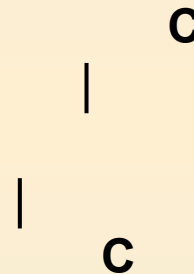
2,3 диметилбутан
