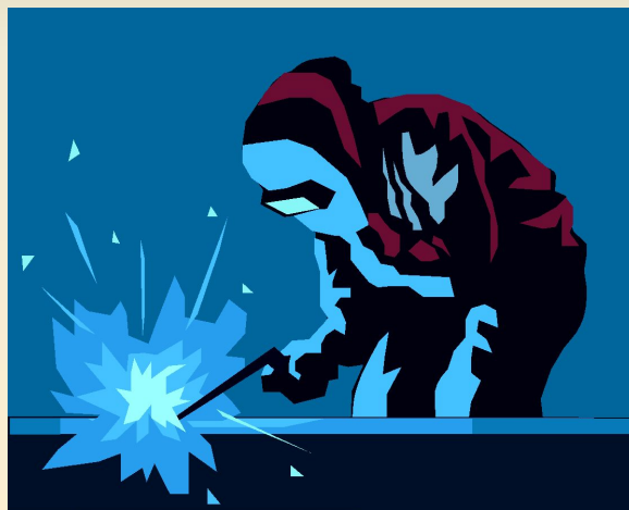
Получение ацетилена
