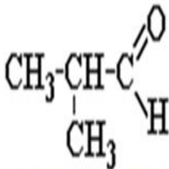
2-метилпропаналь
