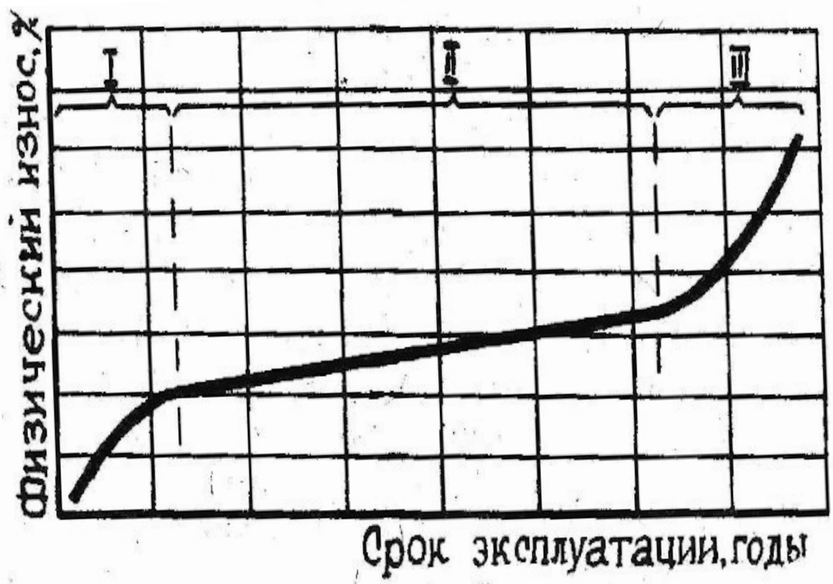
Рис.1 Обобщенный график изменения физического износа объекта в процессе эксплуатации
