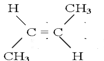
транс-бутен-2
