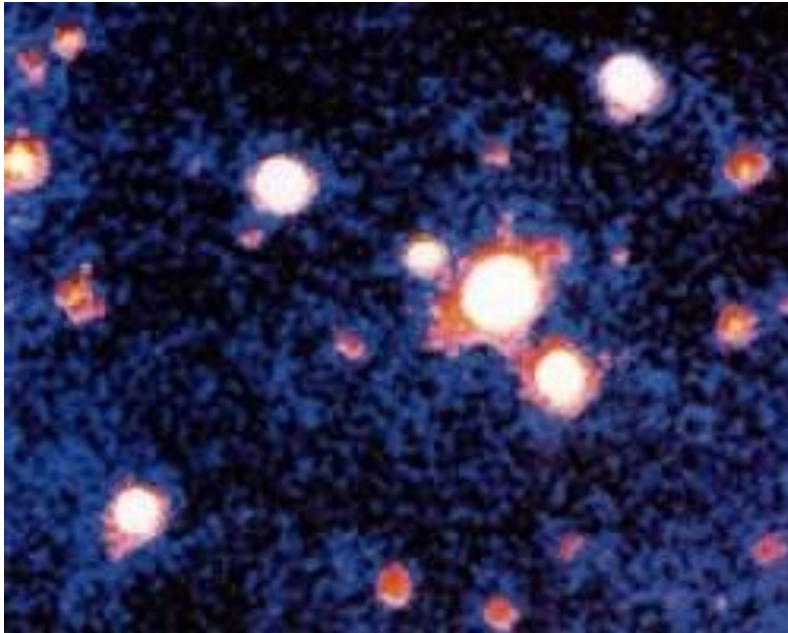
Квазар 3C275
