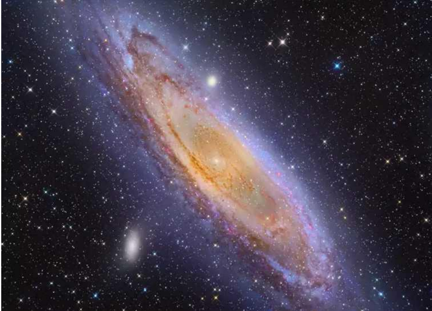
Туманность Андромеды
