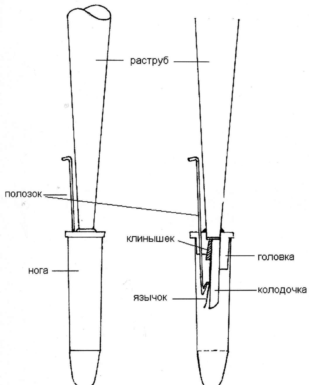
ЯЗЫЧКОВАЯ ТРУБА
