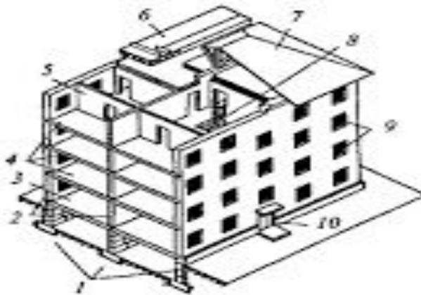
Рис. 3.1. Конструктивные элементы здания:
